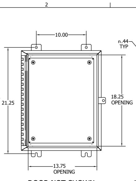
DOOR NOT SHOWN
