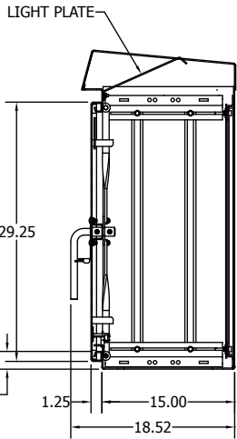
SECTION D-D
